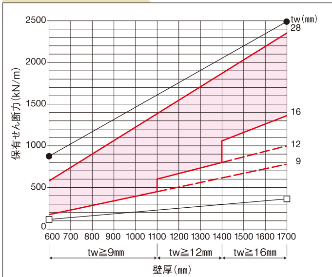
鉛直方向 保有せん断力
