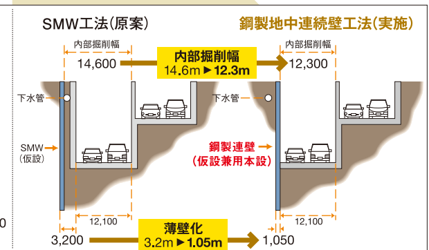
埋設物回避(薄壁化)の適用例
