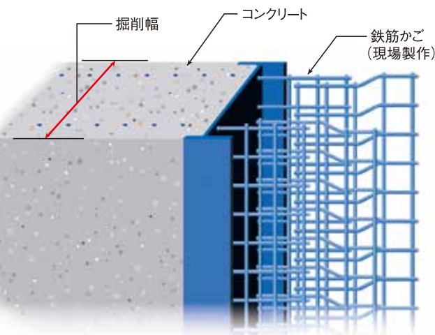
従来工法(コンクリート地中連続壁)
