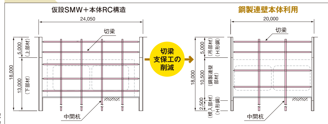
仮設構造例
