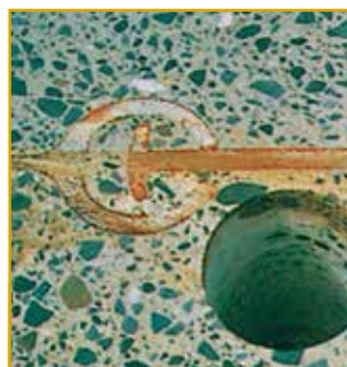
NS-BOX嵌合部 コンクリート充填状況(断面)
