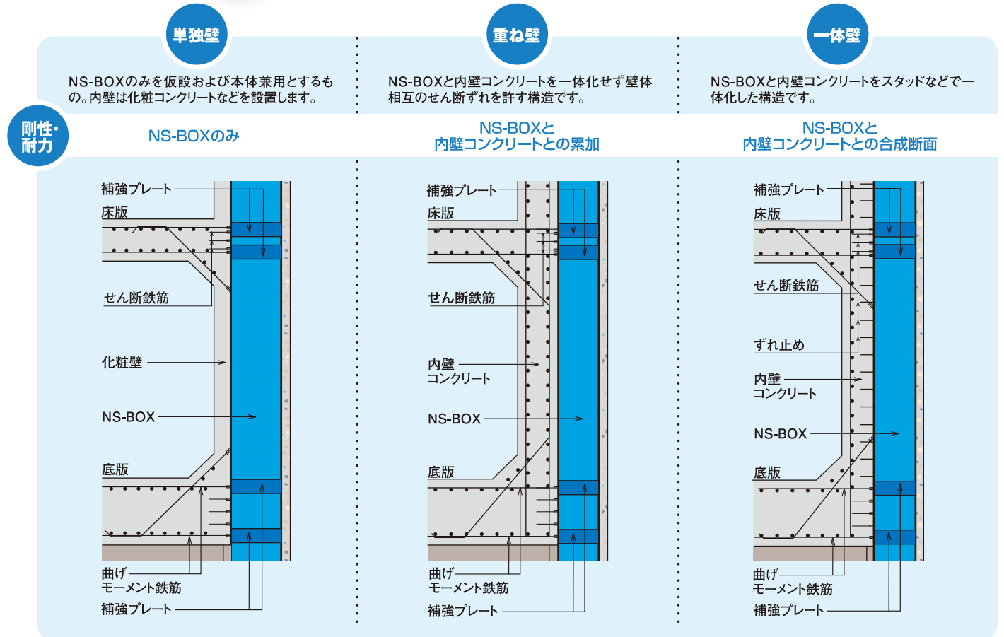
機械継手方式の例
