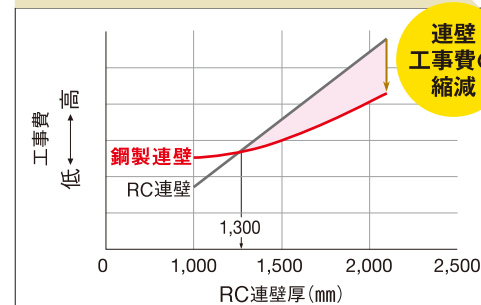
鋼製連壁とRC連壁との経済性比較イメージ
