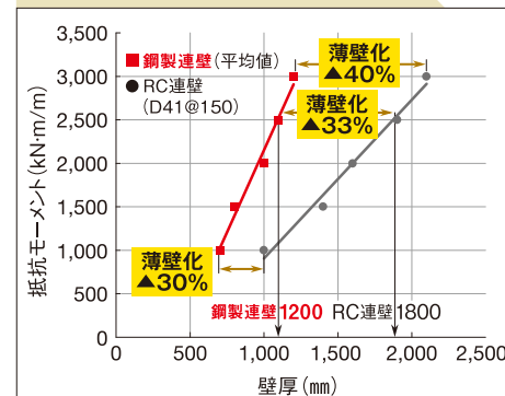
鋼製連壁とRC連壁との壁厚比較例
