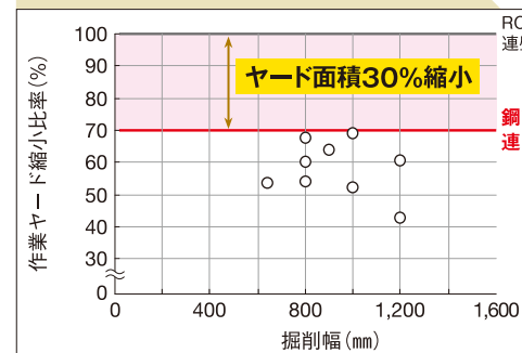
鋼製連壁とRC連壁との現場ヤード比較例
