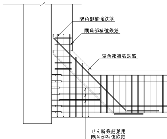
図一参 1.5 隅角部の補強鉄筋
