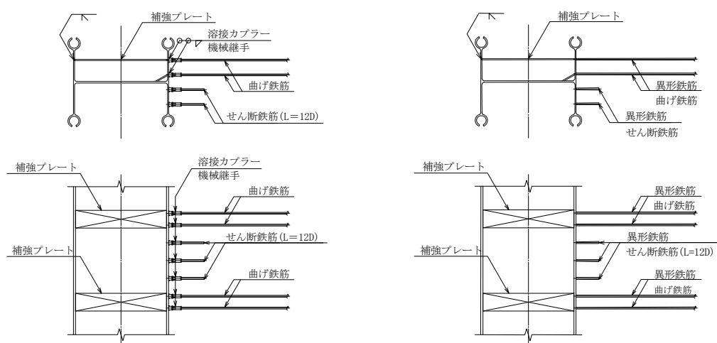
ねじ継手溶接カプラー方式
