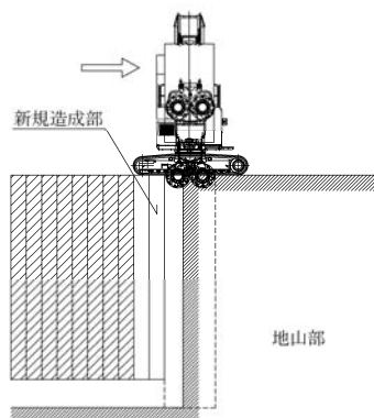
図ー解 3.3.11 標準造成サイクル (2サイクル施工)
