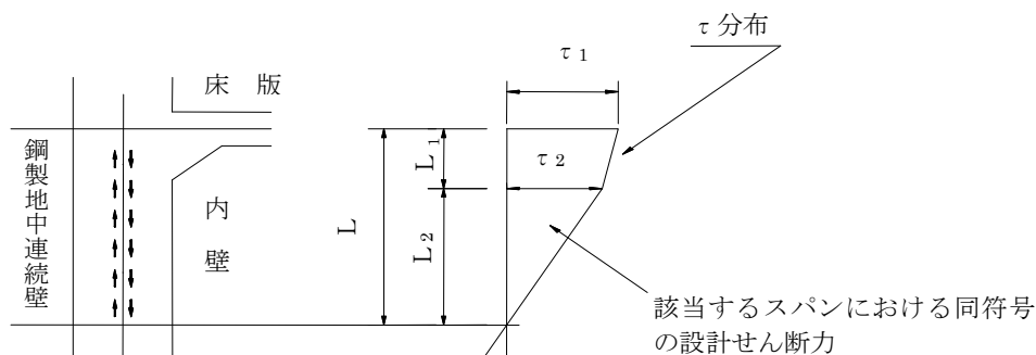
図一解 2.5.15 該当するスパンにおける同符号の設計せん断力
