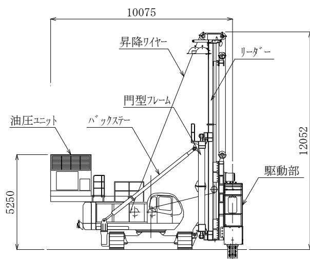
図一参 2.5 TRD-II 型
