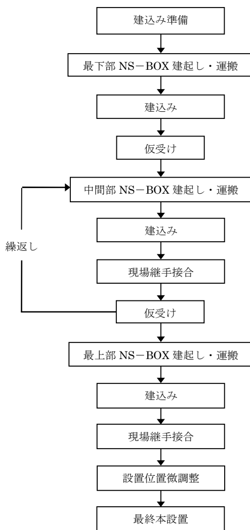
図－解 3. 4. 1 NS-BOX の標準的な建込み手順
