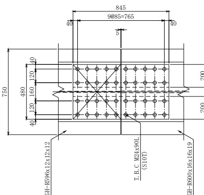
図一解 2.5.9 現場継手の一例
