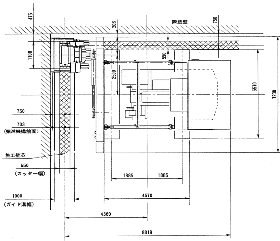
図－参 8.1 T R D 工法機 ( T R D－Ⅲ型) 近接施工平面図
