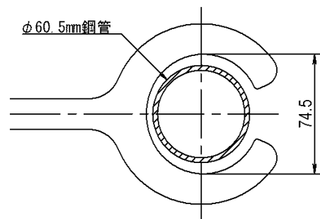
図一解 3. 4. 23 嵌合部 \phi 60.5\text{mm} 防護パイプ
