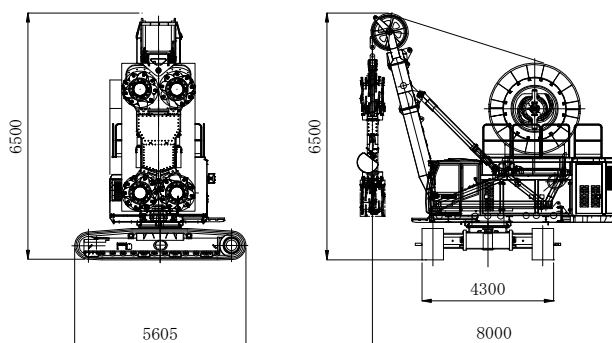
図ー参 3.6 クアトロタイプベースマシン
