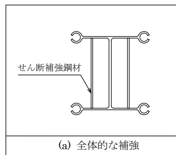
図一解 2.5.4 セン断補強の例
