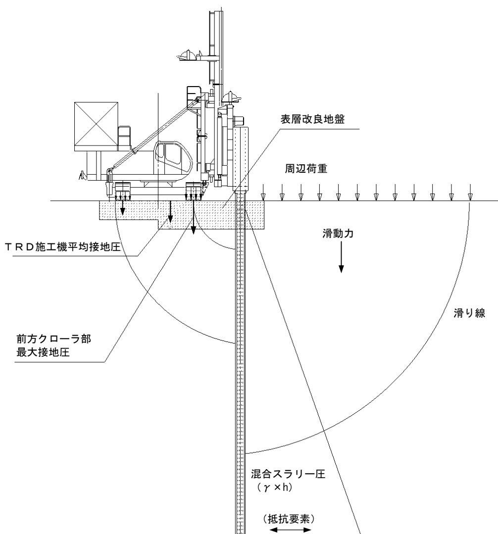
図ー参 2.7 溝壁の安定検討モデル図
