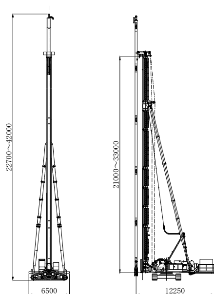
図ー参 3.5 ケリーバータイプベースマシン
