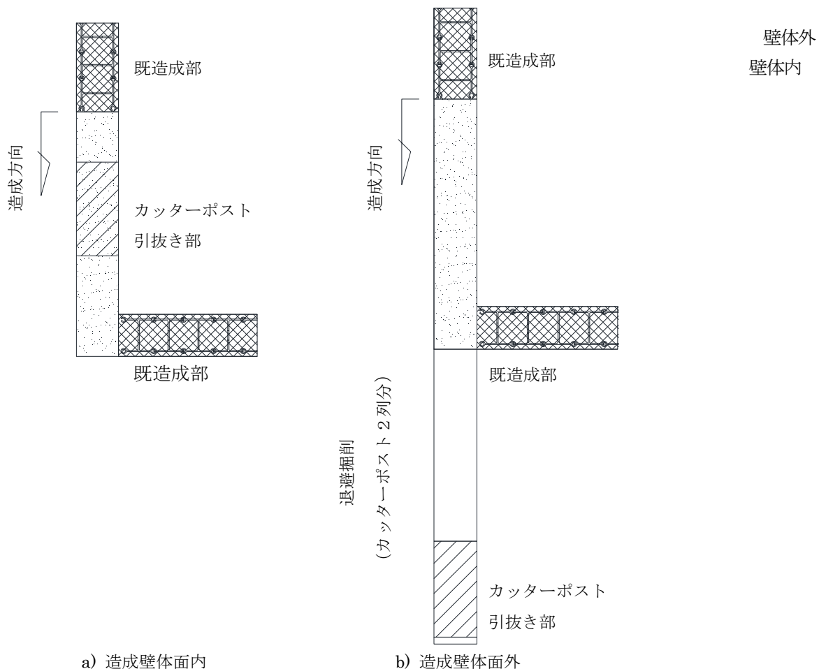
図一解 3.2.8 カッターポスト引抜き位置
