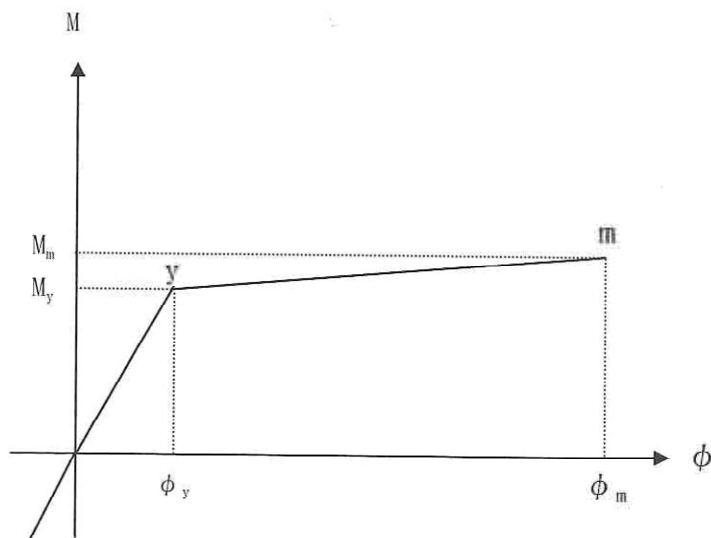
図一参 1.4 曲げモーメントと曲率の関係
