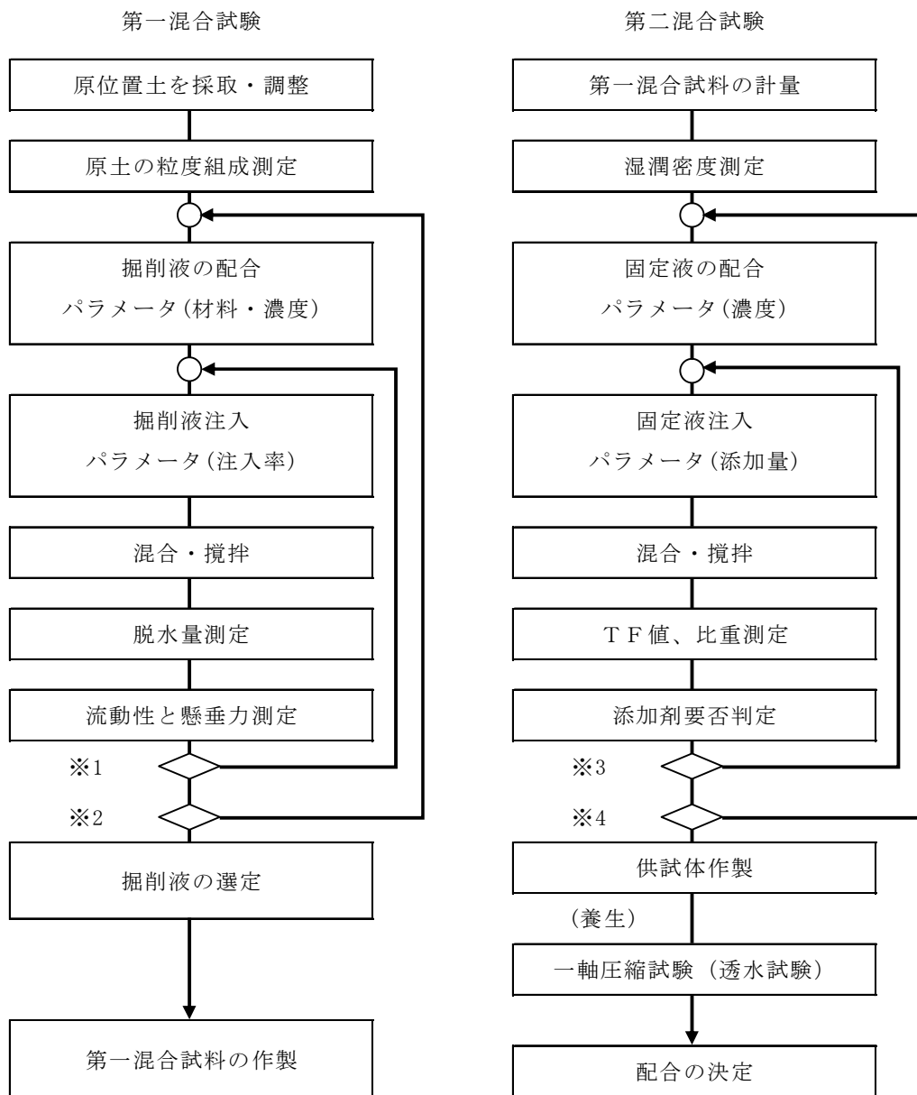
図一解 3.2.4 室内配合試験フロー図
