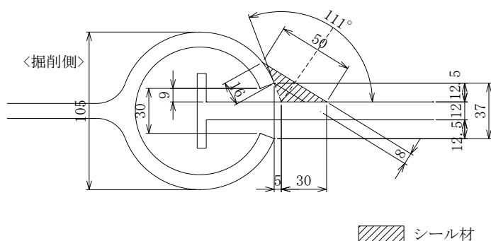
図一参6.10 弾性目地材の塗布形状
