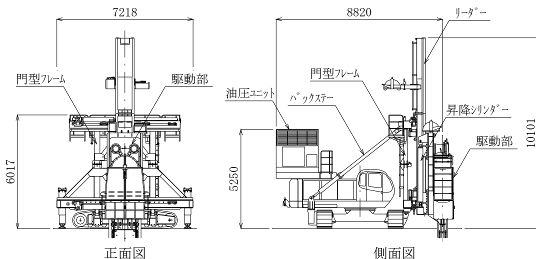
図一解 3.2.2 TRD-III型（標準型）姿図
