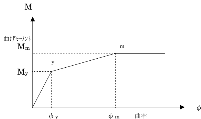
図一解 2.5.6 NS-BOX の曲げモーメントと曲率の関係
