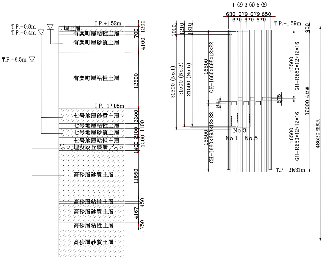
図－参 5.4 観測井配置図（断面図）
