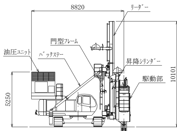
図一参 2.6 TRD-III 型
