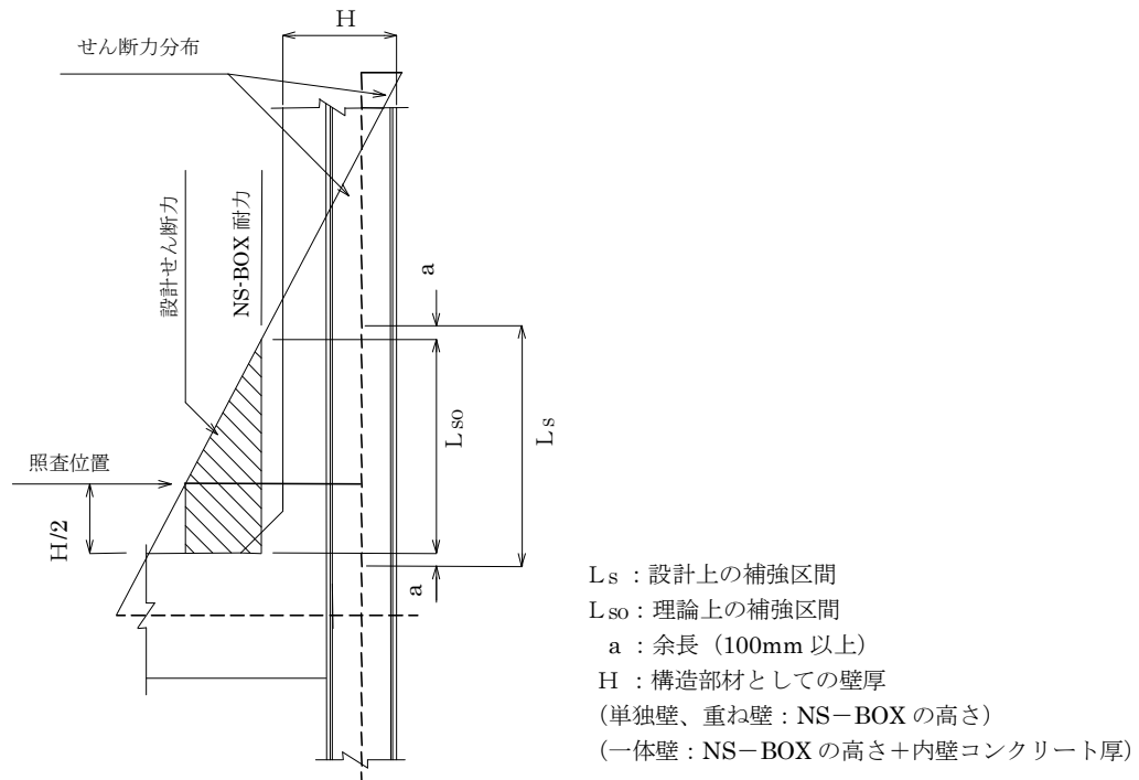
図－解 2.5.5 せん断補強の範囲
