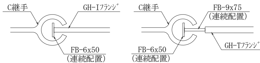
図-1.2.7 嵌合継手
