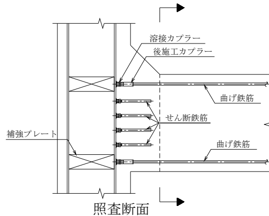
図-参 1.7 せん断鉄筋長
