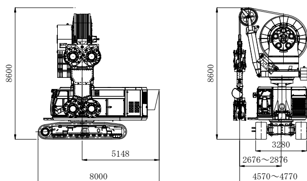
図ー参 3.7 クアトロタイプ(サイドカッター仕様)ベースマシン
